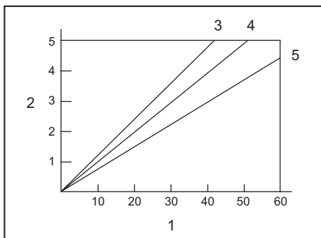
► 1. Fréquence de clouage (fois/min) 2. Sortie d'air du compresseur par minute (CFM (ft³/min)) 3. 0,83 MPa (120 PSIG) 4. 0,66 MPa (95 PSIG) 5. 0,49 MPa (70 PSIG)
