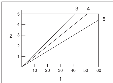
► 1. Frecuencia de clavado (veces/min) 2. Salida de aire del compresor por minuto (CFM: pies cúbicos por minuto (ft 3 /min)) 3. 0,83 MPa (120 PSIG) 4. 0,66 MPa (95 PSIG) 5. 0,49 MPa (70 PSIG)
