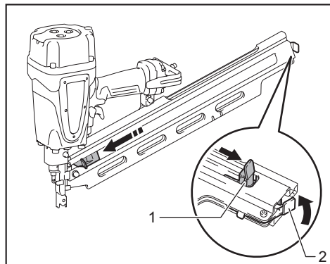
► 1. Palanca pulsadora 2. Palanca de bloqueo
