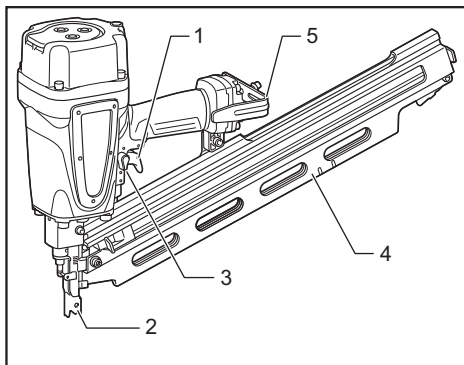
► 1. Gatillo interruptor 2. Elemento de contacto 3. Selector del modo de accionamiento 4. Cartucho 5. Gancho
