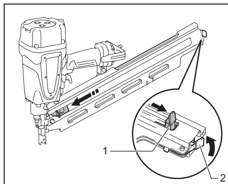
► 1. Levier-poussoir 2. Levier de verrouillage
