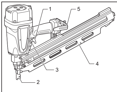
► 1. Gâchette 2. Élément de contact 3. Sélecteur de mode de commande 4. Magasin 5. Crochet
